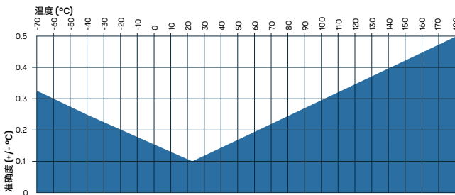
全量程的 HMP5 温度测量准确度
