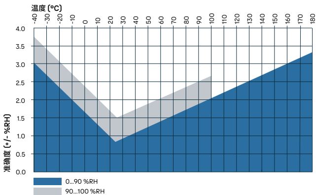
HMP5 湿度测量准确度与温度呈函数关系
