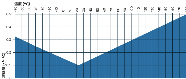
全量程的 HMP4 温度测量准确度
