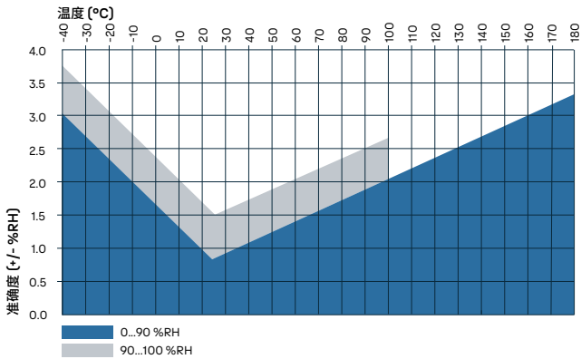
HMP4 湿度测量准确度与温度呈函数关系
