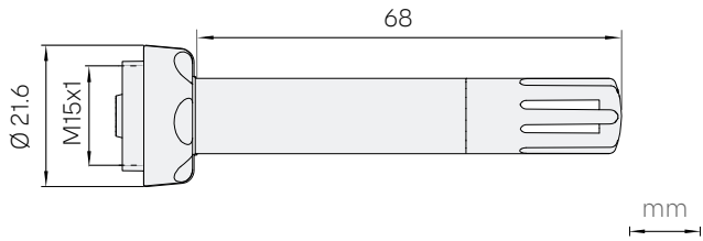
带塑料锁紧衬套的 HMP63 探头尺寸
