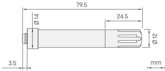
HMP63 探头尺寸
