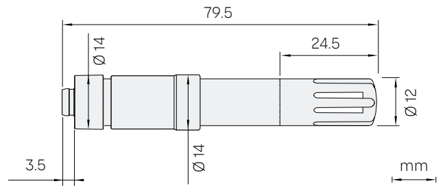
HMP63 和 HMP63T 探头尺寸（带套筒），适用于 CWL100 数据记录仪
